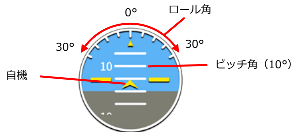
図 19 水平儀の読み方
